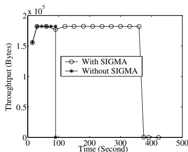
Fig. 7. Throughput in OGSCI scenario.
