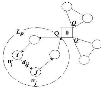
Fig. 1. MCLP
